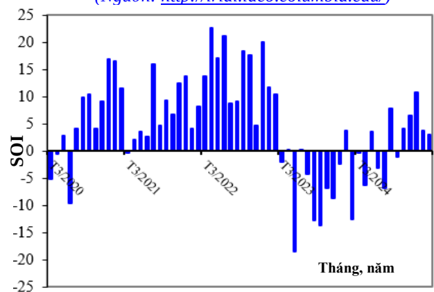
Hình 1.3. Diễn biến chỉ số SOI (3/2020 - 2/2025)
